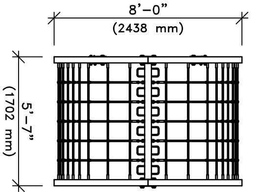
TOP VIEW SCALE: NONE
